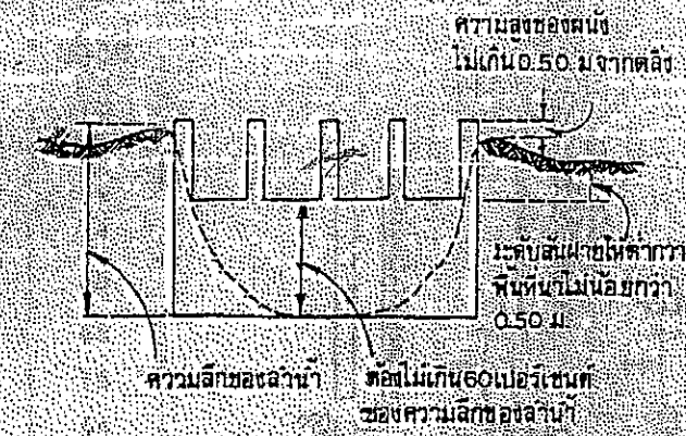
การออกแบบฝาย
