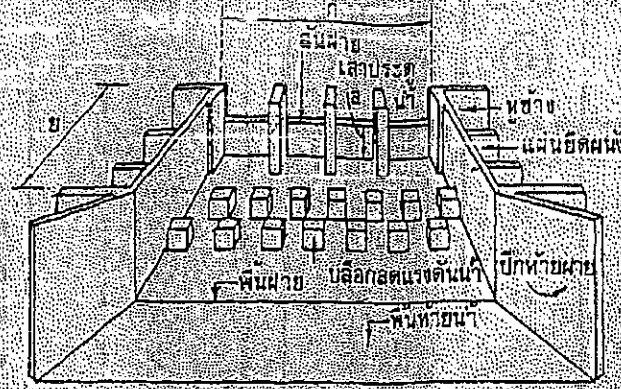
แบบฝายมาตรฐาน มข. 2527
