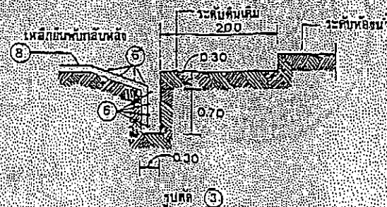
การเทคอนกรีตผนังฝั่งดิน
