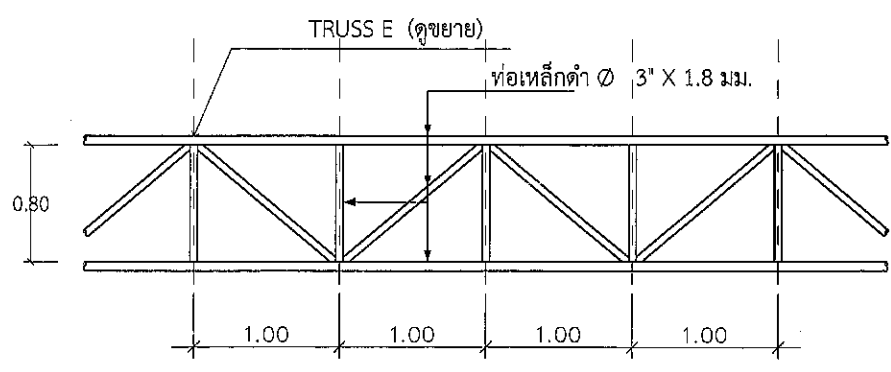
แบบขยาย TRUSS B SCALE 1: 50
